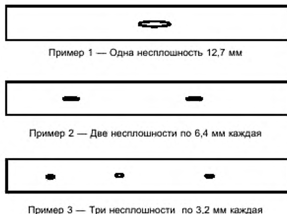
Рисунок 9 — Примеры схем максимальных распределений обнаруженных несплошностей типа удлиненных шлаковых включений на рентгенограммах
